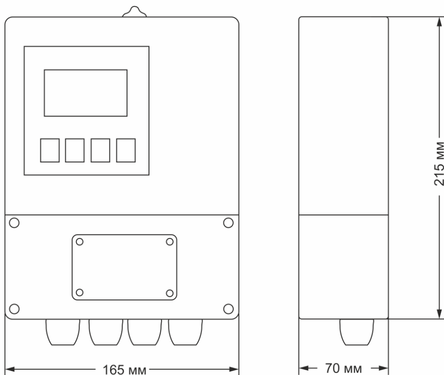
Рис.6. Схема раздельного электромагнитного расходомера
