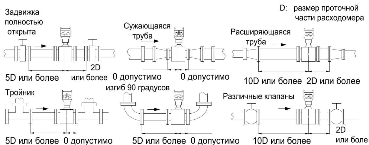
Рис.4. Требования к прямолинейным участкам
